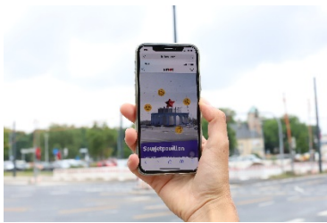
20211129_smac_AppReleaseAndroid_Bild01.jpg
